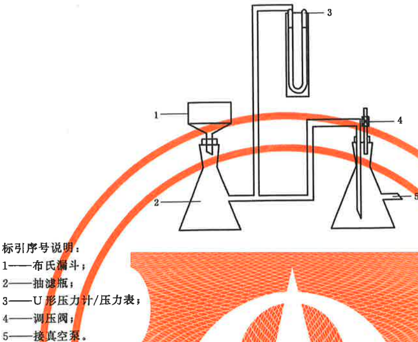
图 1 保水率测定仪结构示意图
